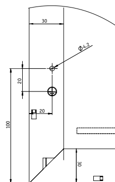
Detail aanzicht - aardingsgat
