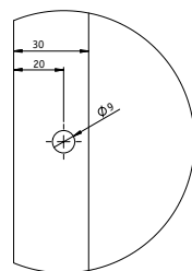
Detail aanzicht - montagegat
