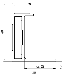
Frameprofiel
